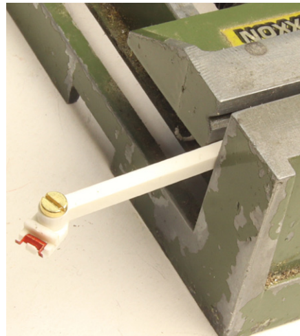
Mit 2K-Kleber (z. B. UHU plus schnellfest) an die Pufferhülse kleben. Nach dem Aushärten Klebehilfe nach unten drücken und entfernen.
